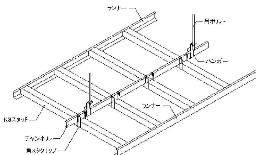
図1-2 天井下地 基本構成図
