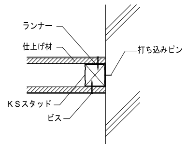
a 断面図
